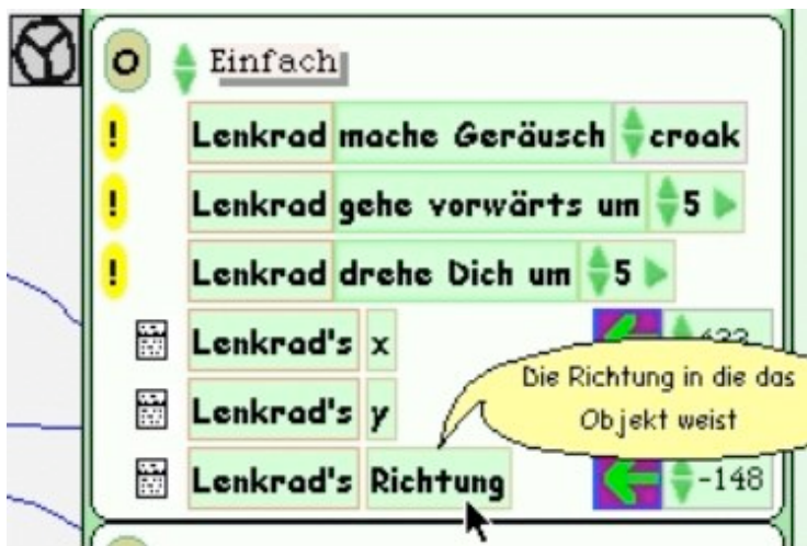
Abbildung 11: Auch Variablen können aus den Vorlagen kopiert werden
